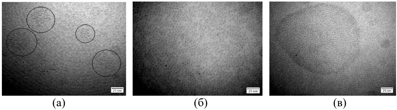
Рис.1. ПЕМ-зображення нанокмпозитних плівок PVK-CdZnSeS/ТОРО товщиною 80-100 нм при концентрації НЧ: (а) 4 об. %; (б) 39 об.%; (в) 46 об.%.
