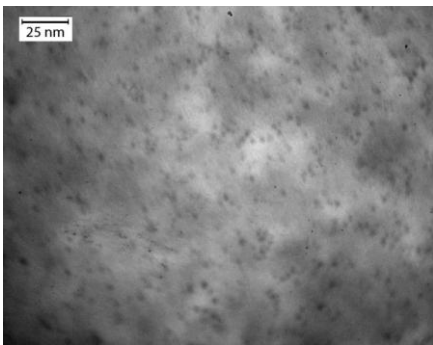
Рис.3. ПЕМ-зображення ПНН PFO-CdZnSeS/ТОРО ( C_{\text{НЧ}} = 42 об.%)
