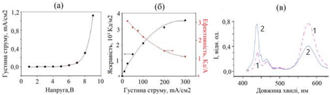
Рис. 11. Вольт-амперна характеристика (а) та залежність яскравості і ефективності за струмом ЕЛ від щільності струму (б) для структури ІТО/PEDOT:PSS/PFO+НЧ/ Bu-PBD/Al (в) спектр електролюмінесценції структури ІТО/PEDOT:PSS/PFO/НЧ/ Bu-PBD /Al (1) та ІТО/PEDOT:PSS/PFO+НЧ/ Bu-PBD /Al (2).
