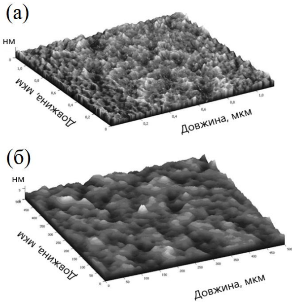
Рис.2. АСМ-зображення фрагменту поверхні плівки PVK (товщиною 80 нм) та ПНН PVK-CdZnSeS/ТОРО ( C_{\text{НЧ}} = 17 об.%, товщина 80 нм) на ІТО підкладці.
